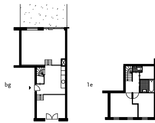
woningtype 4B - GBO: 93m 2
