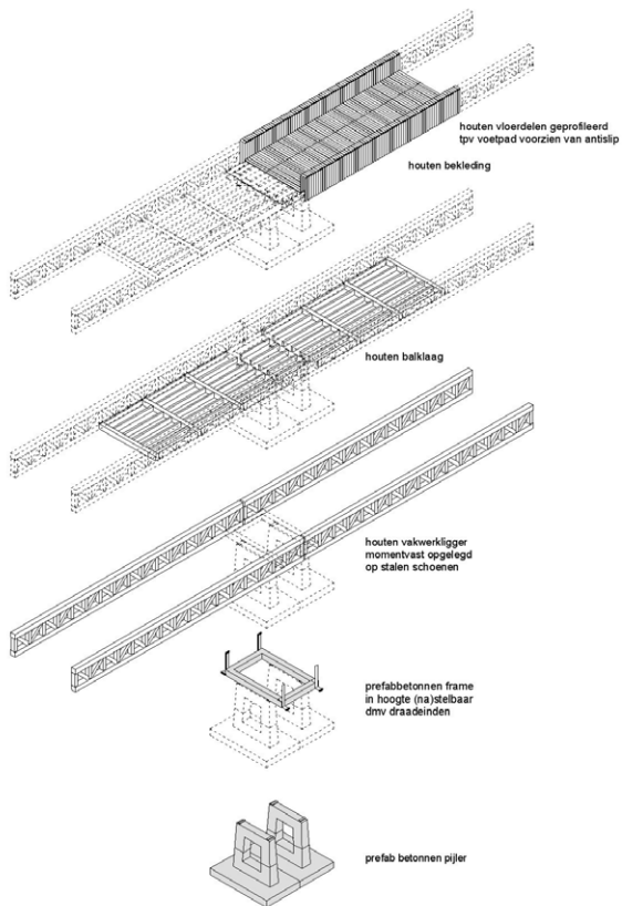
Axonometrie constructie principe
