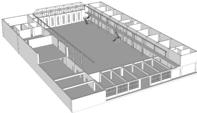
3D schema: casco, vloervlakken, nieuwe toevoegingen
